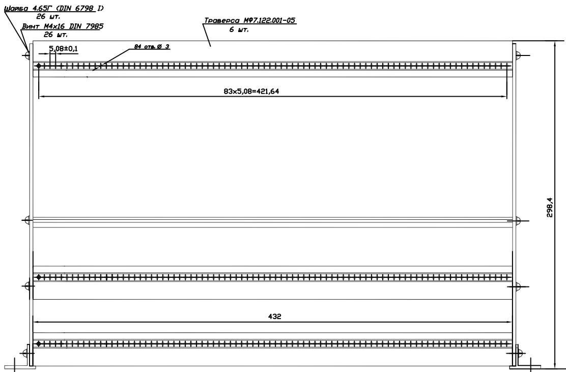
Рисунок 1 - КАРКАС 6U МФ4.122.089-05. ГАБАРИТНЫЕ И ПРИСОЕДИНИТЕЛЬНЫЕ РАЗМЕРЫ.
